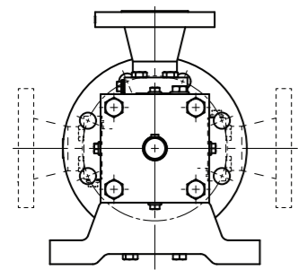
SNAH 前视图
