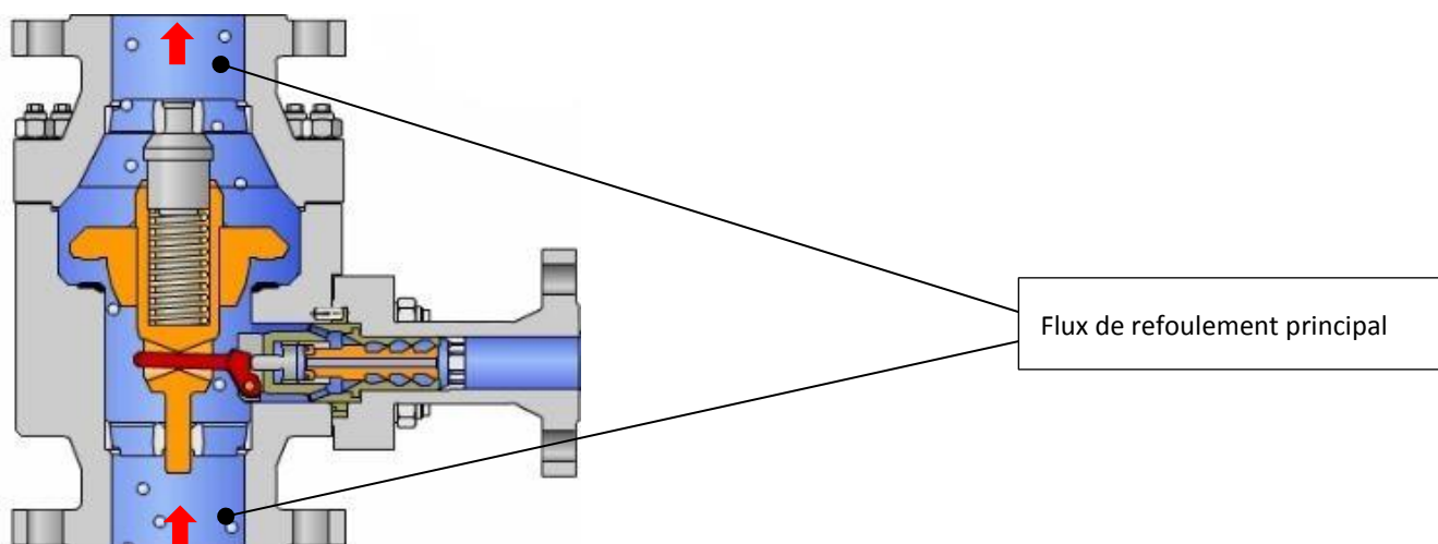
Figure 4 Robinetterie TDM avec dispositif antiretour conique ouvert et écoulement libre en cours de fermeture (point de commutation)
