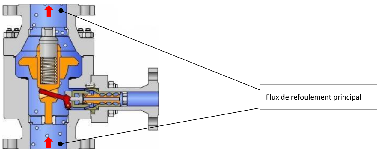
Figure 5 Robinetterie TDM avec dispositif antiretour conique ouvert à la hauteur de course maximale et écoulement libre fermé
