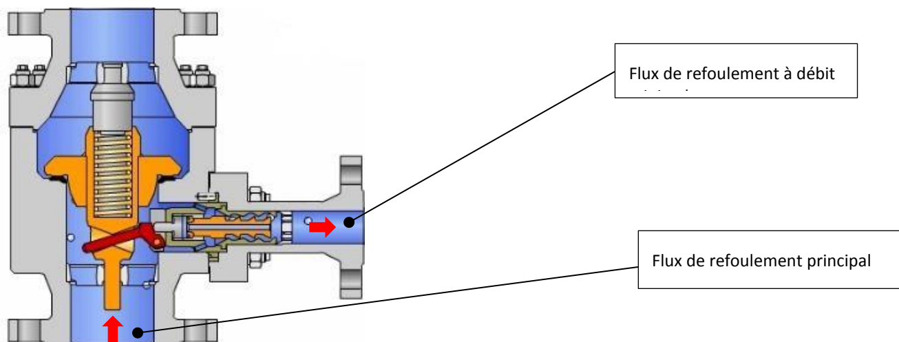
Figure 3 Robinetterie TDM avec dispositif antiretour conique fermé et écoulement libre ouvert
