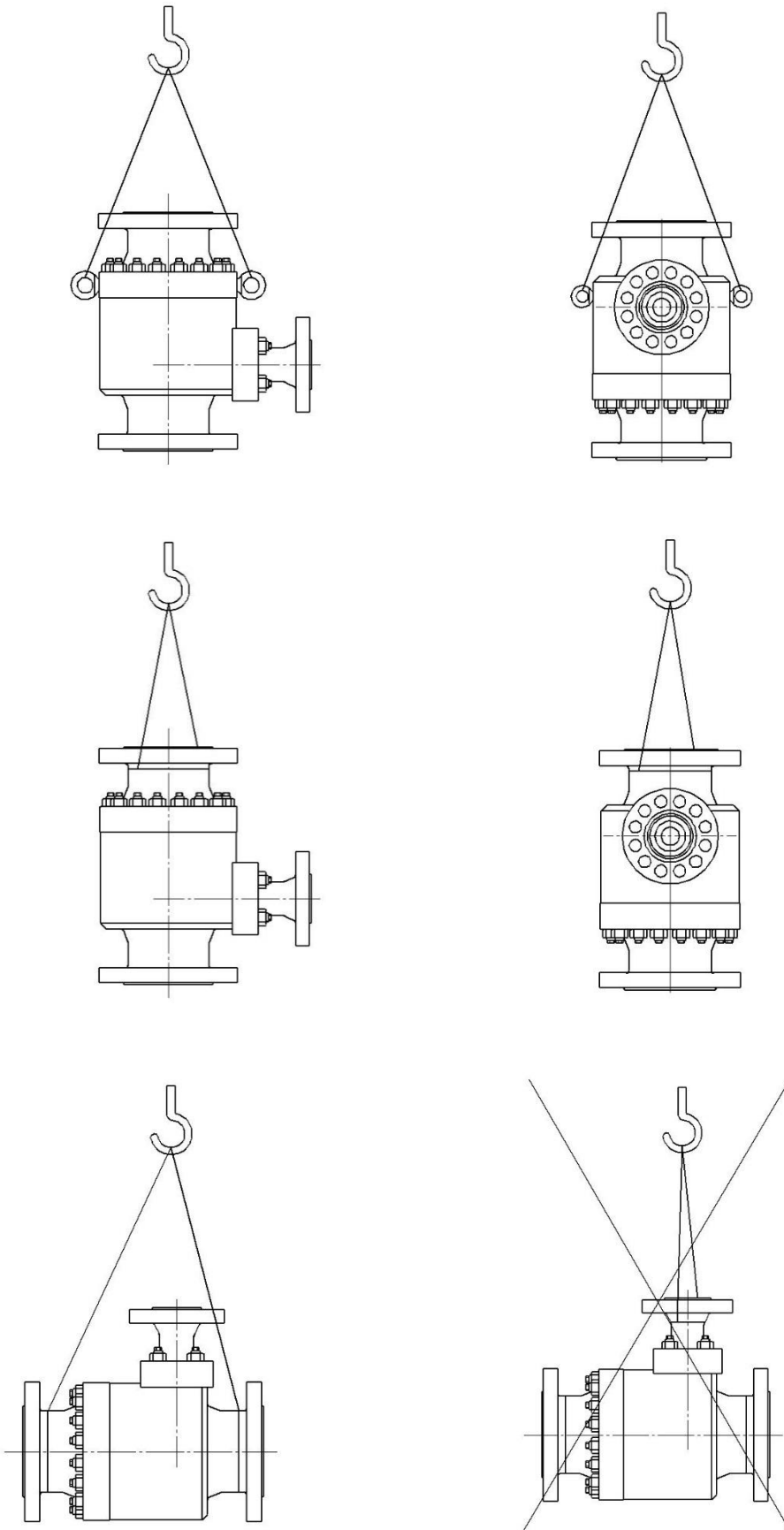
Figura 10 Ejemplo que ilustra las opciones de manipulación durante la instalación de la válvula
