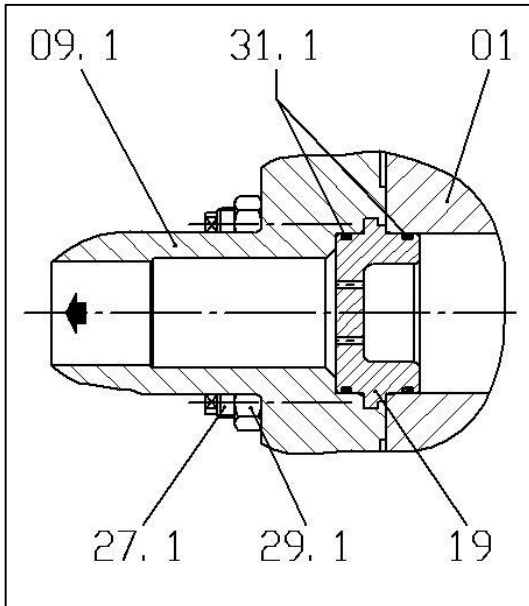
Figura 12 Tubuladura de arranque manual tipo TDL con lista de piezas
