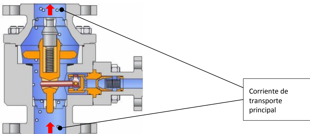
Figura 4 Válvula TDL con cono de retención abierto y rueda libre cerrándose (punto de conmutación)
