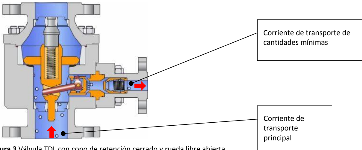
Figura 3 Válvula TDL con cono de retención cerrado y rueda libre abierta
