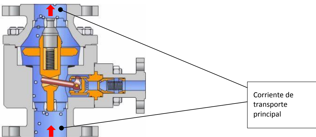
Figura 5 Válvula TDL con cono de retención abierto en altura de elevación máxima y rueda libre cerrada
