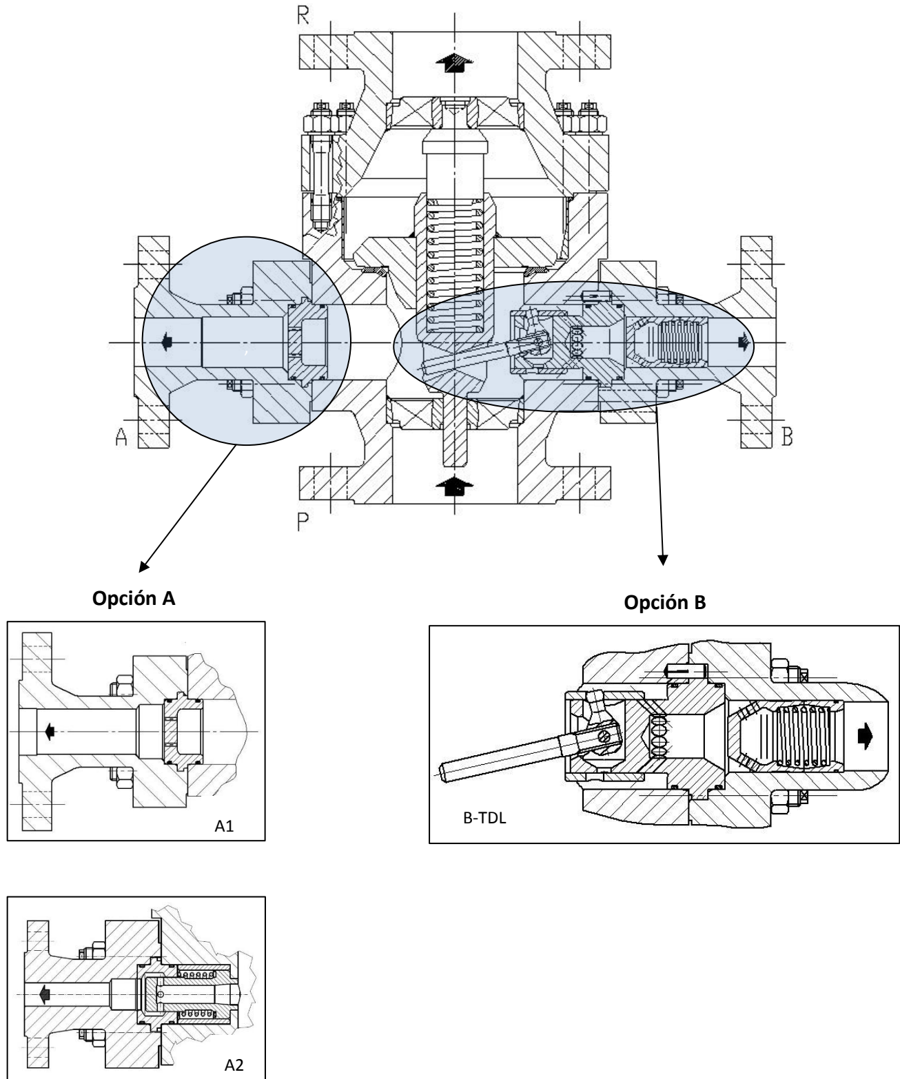
Figura 8 Válvula tipo TDL con diferentes tubuladuras de arranque A1 y A2 (izquierda) y B-TDL (derecha)
