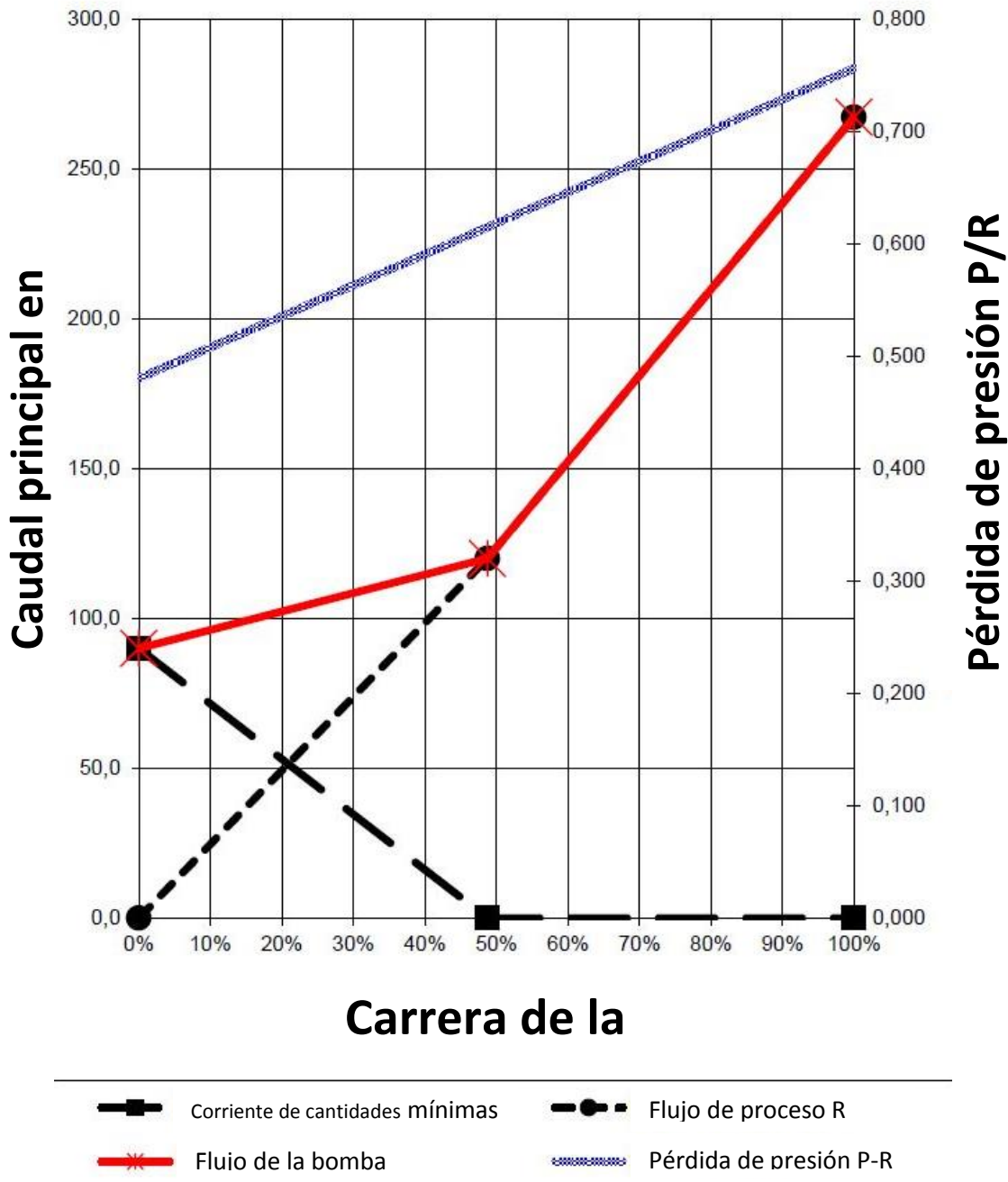
Figura 6 Curva característica de una válvula de cantidades mínimas del tipo TDL
