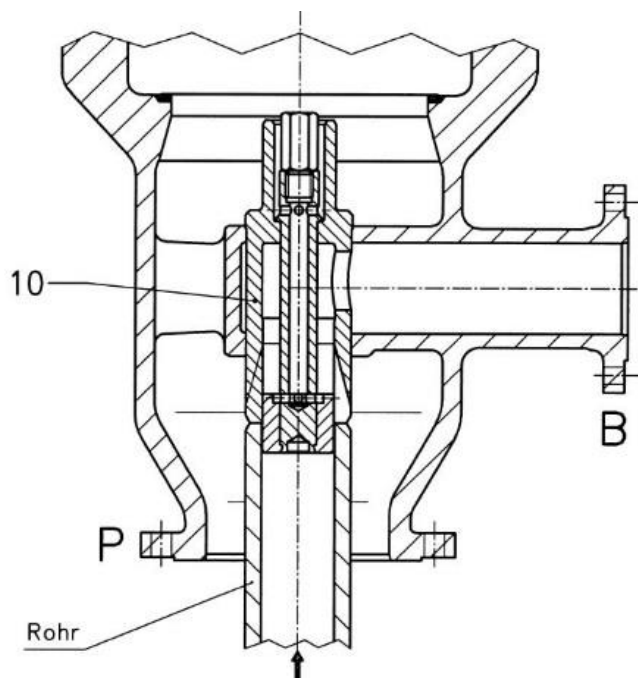
Figure 11 Démontage de la pièce rapportée d'écoulement libre (Pos. 10 – 13)
