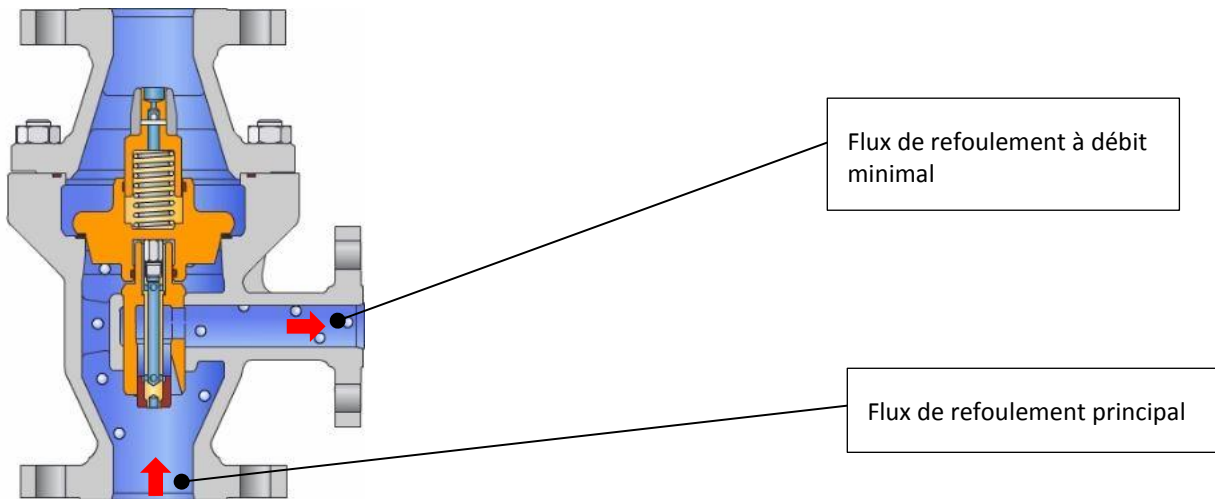
Figure 3 Robinetterie SUL avec dispositif antiretour conique fermé et écoulement libre ouvert
