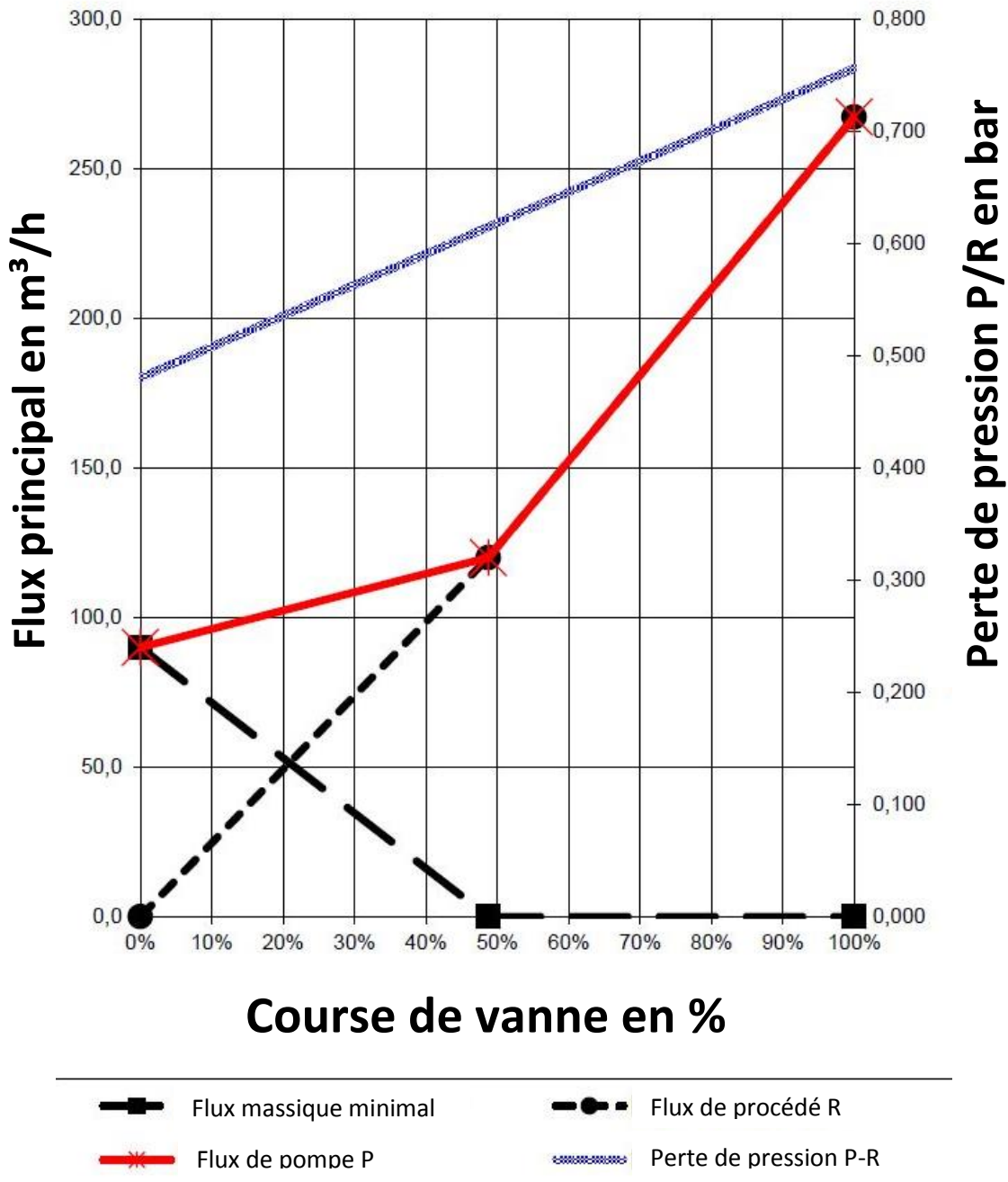
Figure 6 Courbe caractéristique d'une robinetterie à débit minimal de type SUL
