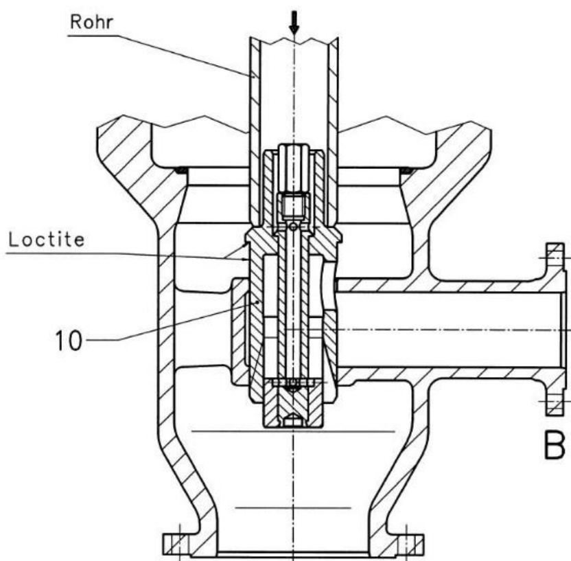
Figure 12 Montage de la pièce rapportée d'écoulement libre (pos. 10 – 13)
