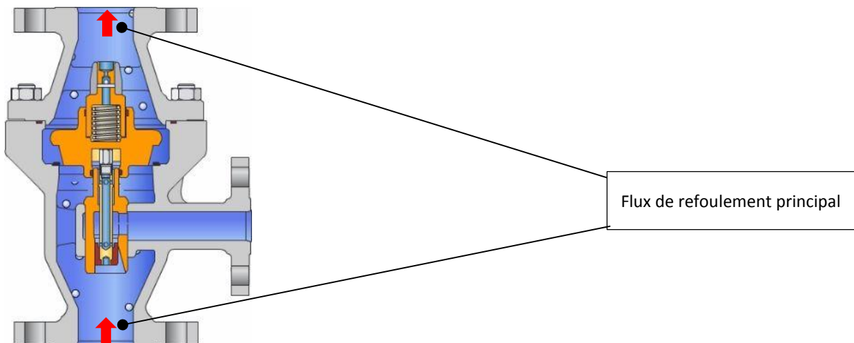
Figure 5 Robinetterie SUL avec dispositif antiretour conique ouvert à la hauteur de course maximale et écoulement libre fermé
