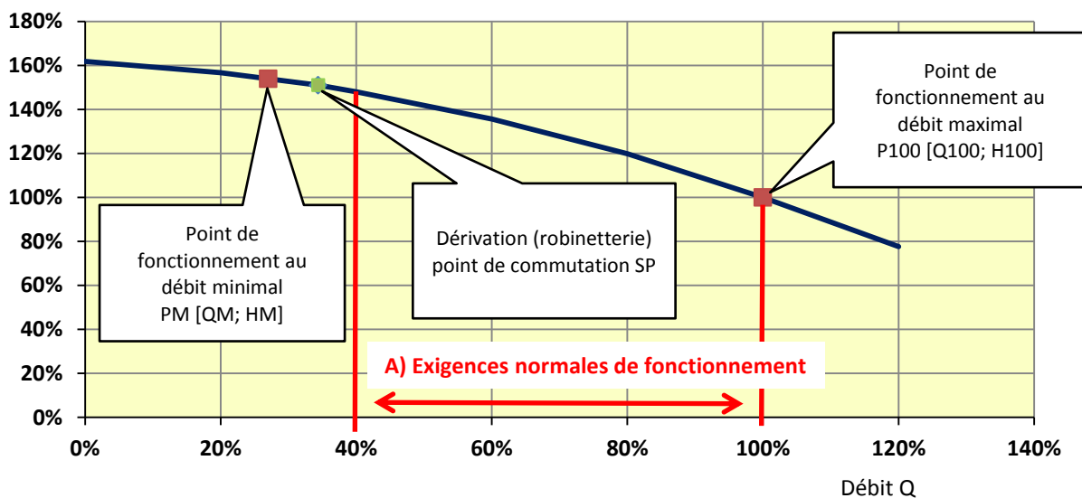
Figure 7 Exigence normale de fonctionnement
