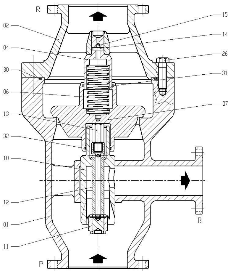
Figure 1 Plan en coupe et liste de pièces de la robinetterie de type SUL sans fonction antiretour (exemple)
