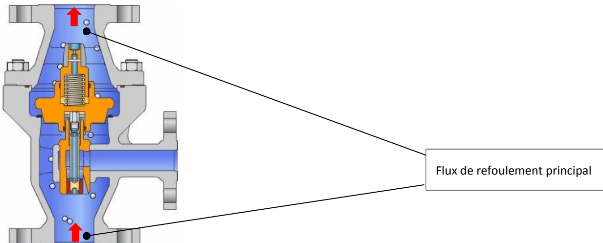
Figure 4 Robinetterie SUL avec dispositif antiretour conique ouvert et écoulement libre en cours de fermeture (point de commutation)
