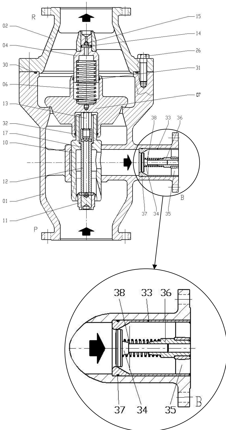
Figure 2 Plan en coupe et liste de pièces de la robinetterie de type SUL avec fonction antiretour (exemple)
